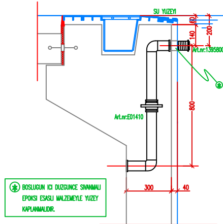
DETAY NO:5 VAKUM BETON GECİS
