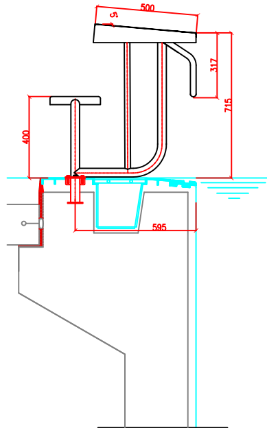
ATLAMA PLATFORMU YERLEŞİM DETAYI (Teslimat Çerçevesinde değildir)
