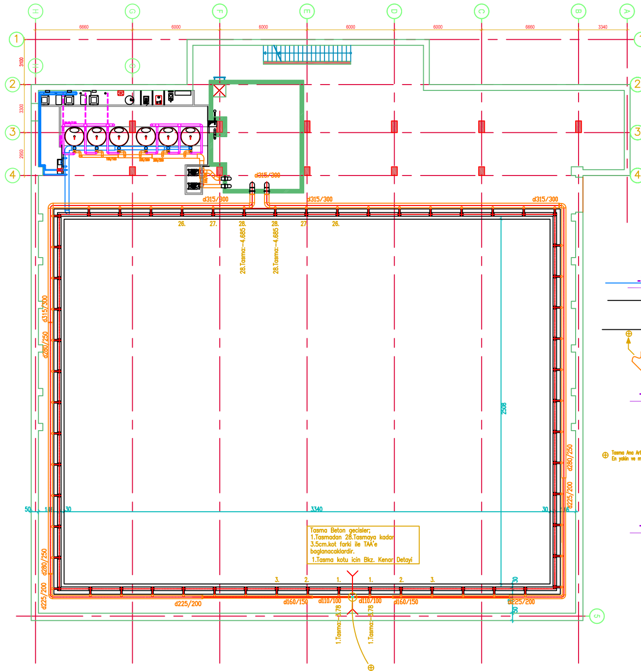
HAVUZ TASMA ANA ARTEL TESİSATI YERLEŞİMİ
