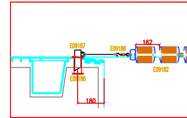
KULVAR SEPERATÖRÜ YERLEŞİM DETAYI
