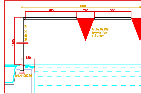
GERİ DÖNÜS İKAZ SETİ YERLEŞİM DETAYI
