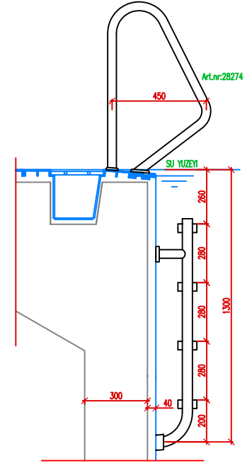
DETAY NO:6 MERDİVEN YERLESİM PLANI
