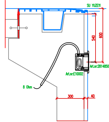
DETAY NO:3 SUALTI HOPERLÖRÜ YERLESİMİ
