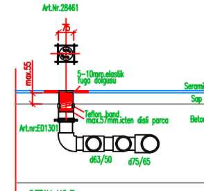
DETAY NO:7 DİP BESLEME DETAYI
