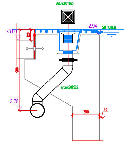
DETAY NO:1 BETON GECİS ELEMANI
