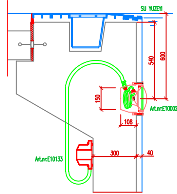
DETAY NO:2 SUALTI PROJİKTÖRÜ YERLESİMİ
